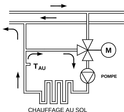
Vanne mélangeuse
